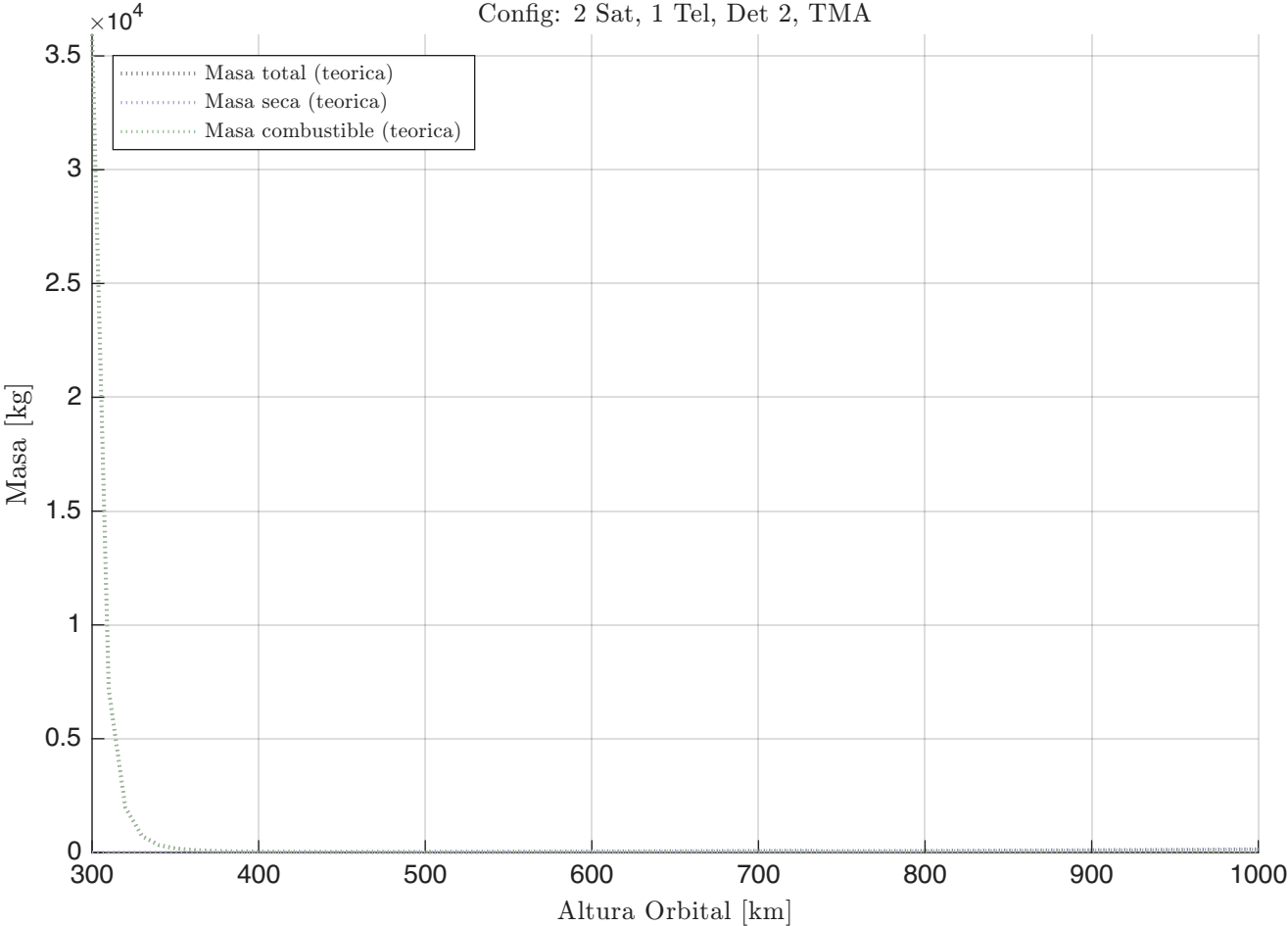
Desglose de Masas vs. Altura Config: 2 Sat, 1 Tel, Det 2, TMA
